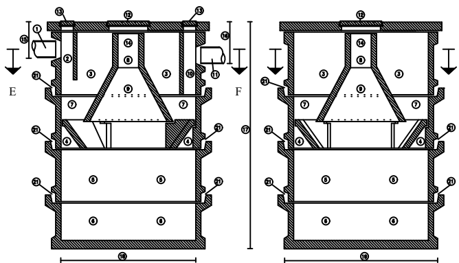
SEZIONE C-D
