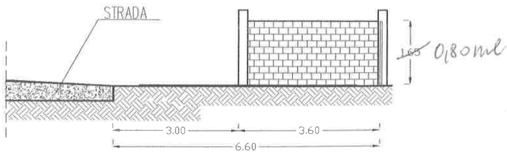
SEZIONE VARCO
