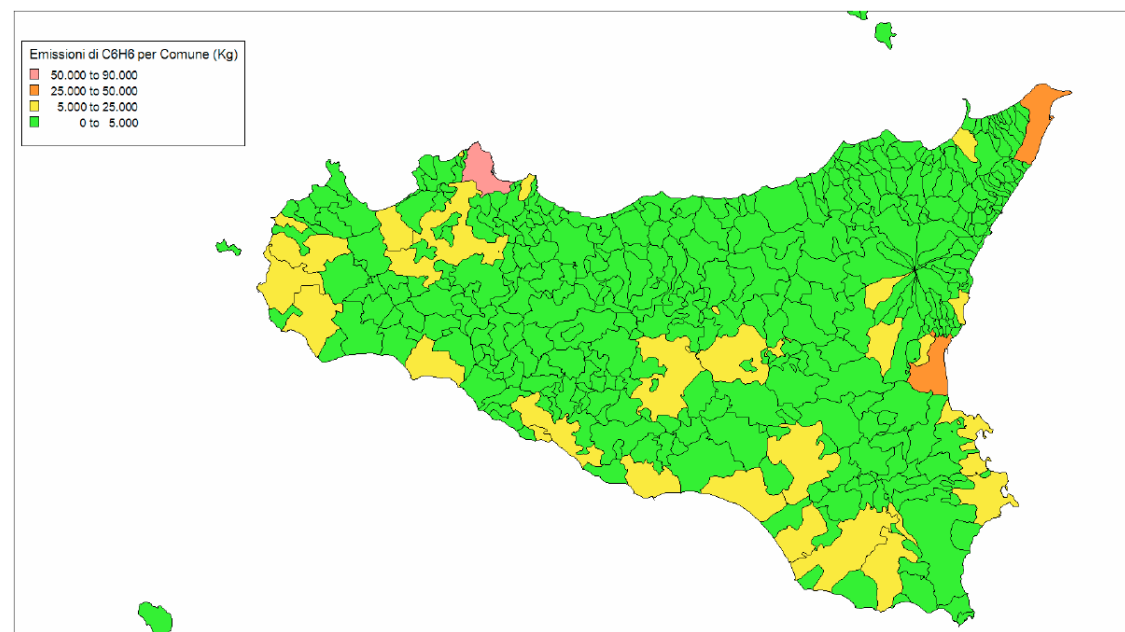
Emissioni di C 6 H 6 distribuite per Comune, anno 2007
