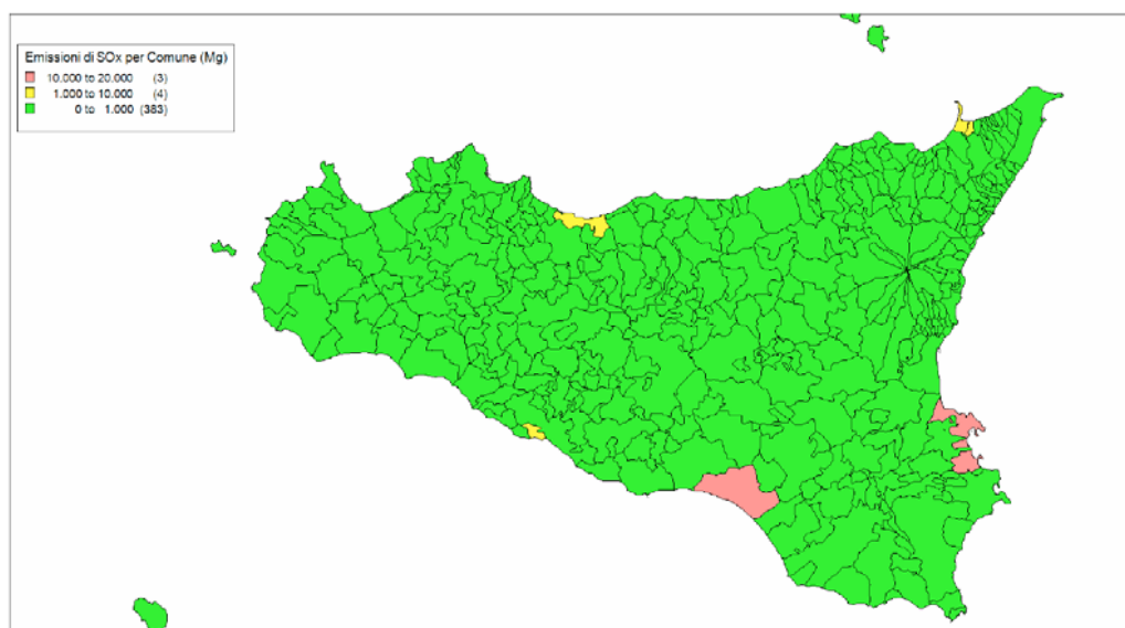
Emissioni di SOx distribuite per Comune, anno 2007
