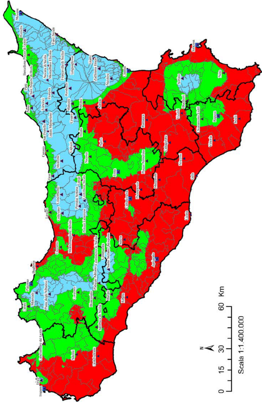
Carta 3.1 –Indice di aridità (ETP/P)
