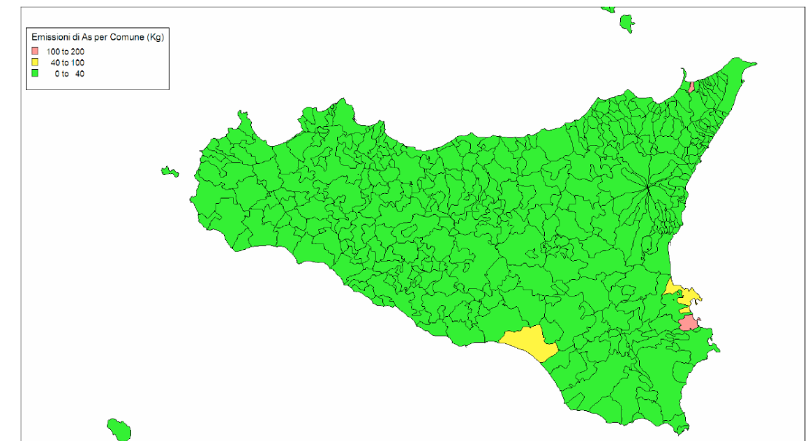
Emissioni di As distribuite per Comune, anno 2007
