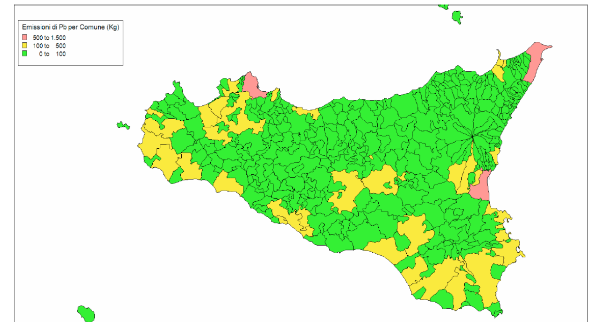
Emissioni di Pb distribuite per Comune, anno 2007
