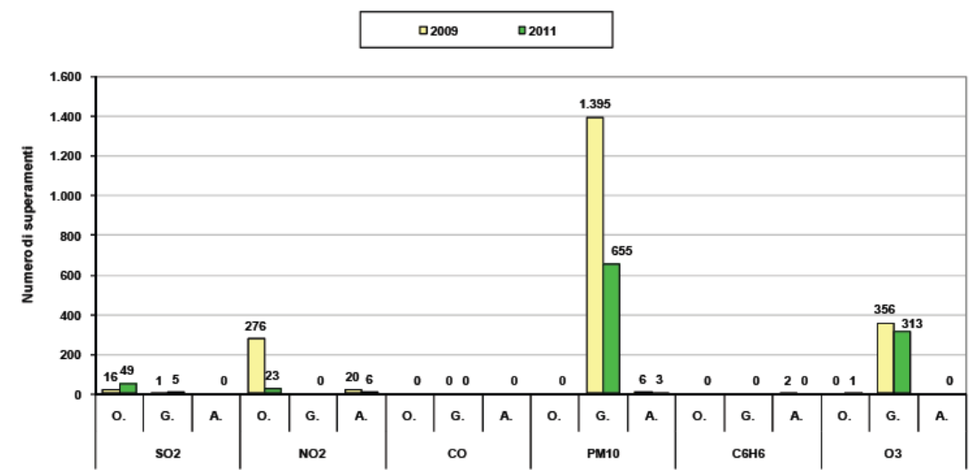
Andamento dell'indicatore "Numero di superamenti dei valori soglia nell'atmosfera di inquinanti pericolosi per la salute umana (CO, NO 2 , PM 10 , C 6 H 6 , SO 2 , O 3 )" nel periodo 2009- 2011
