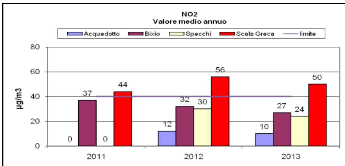
Grafico 9 : NO 2 Valore medio annuale
