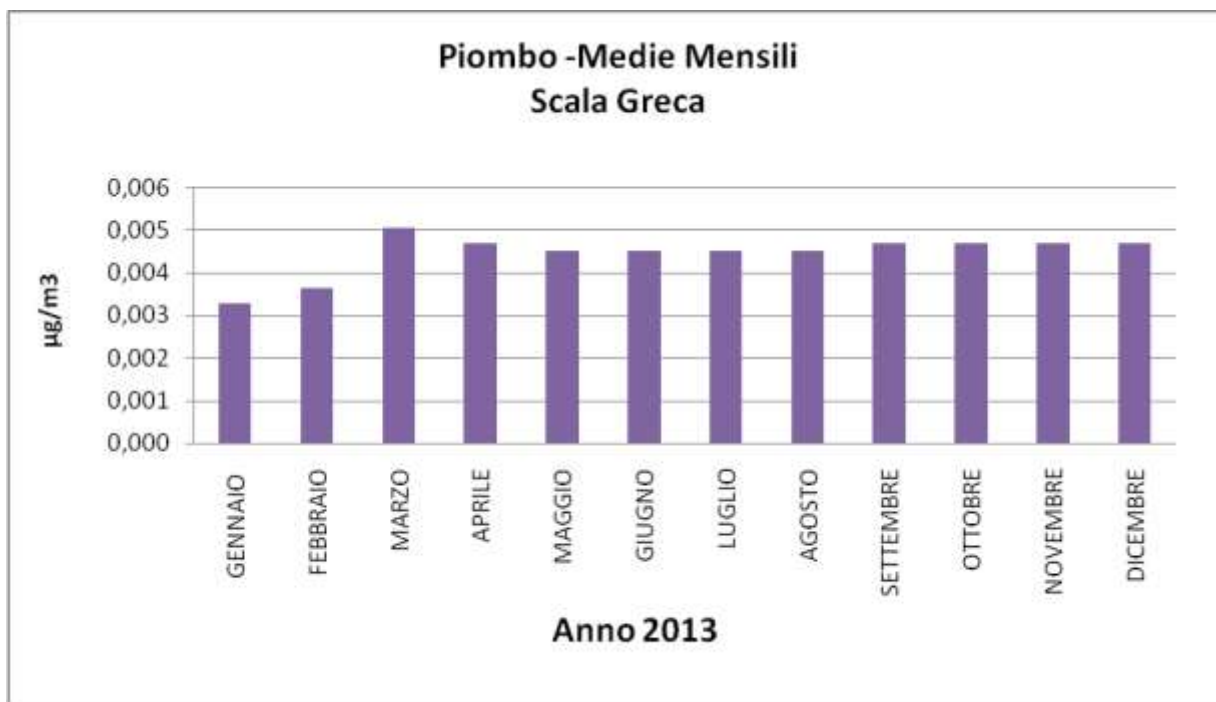
Grafico 23 : Piombo- Valore medio mensile
