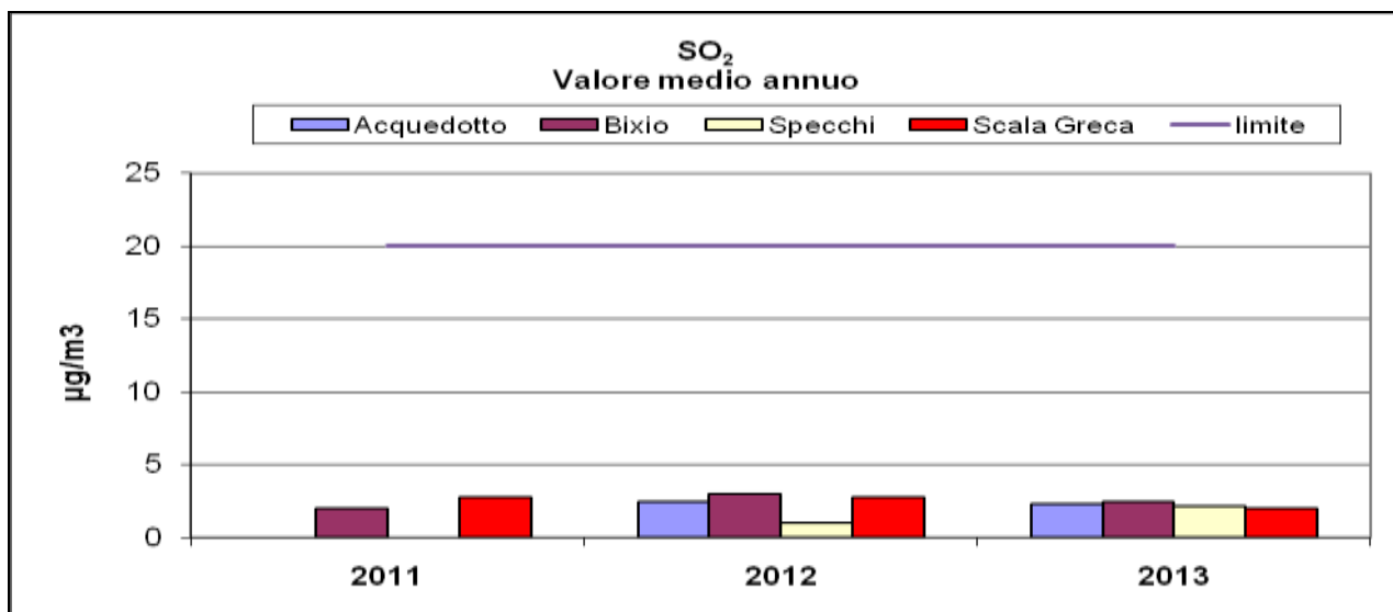
Grafico 6 : SO 2 valori medio annuale
