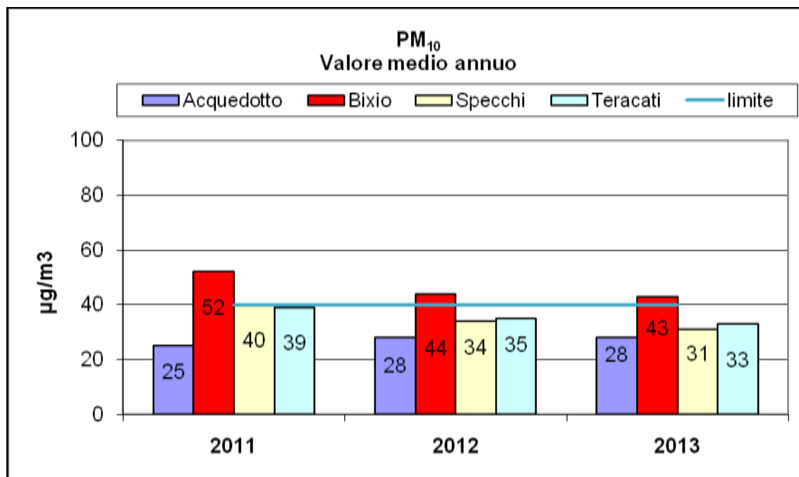
Grafico 18 : PM10: Valore medio annuale
