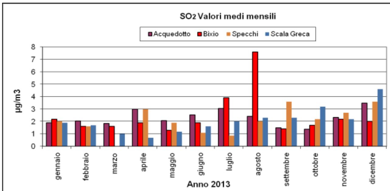
Grafico 7 : SO 2 valori medi mensili
