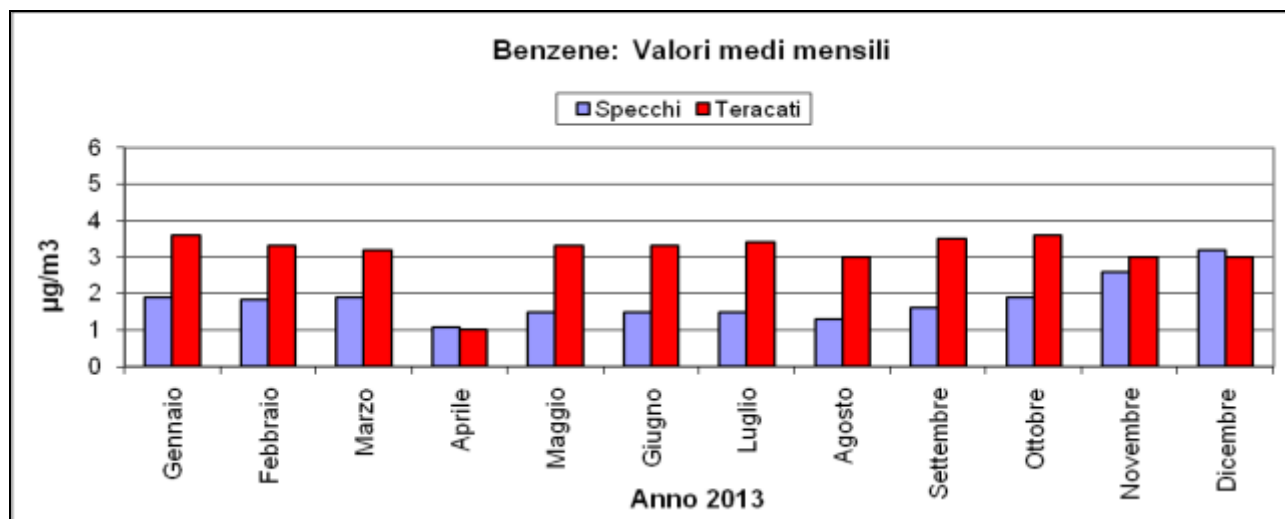
Grafico 21 : Benzene Valore medio mensile
