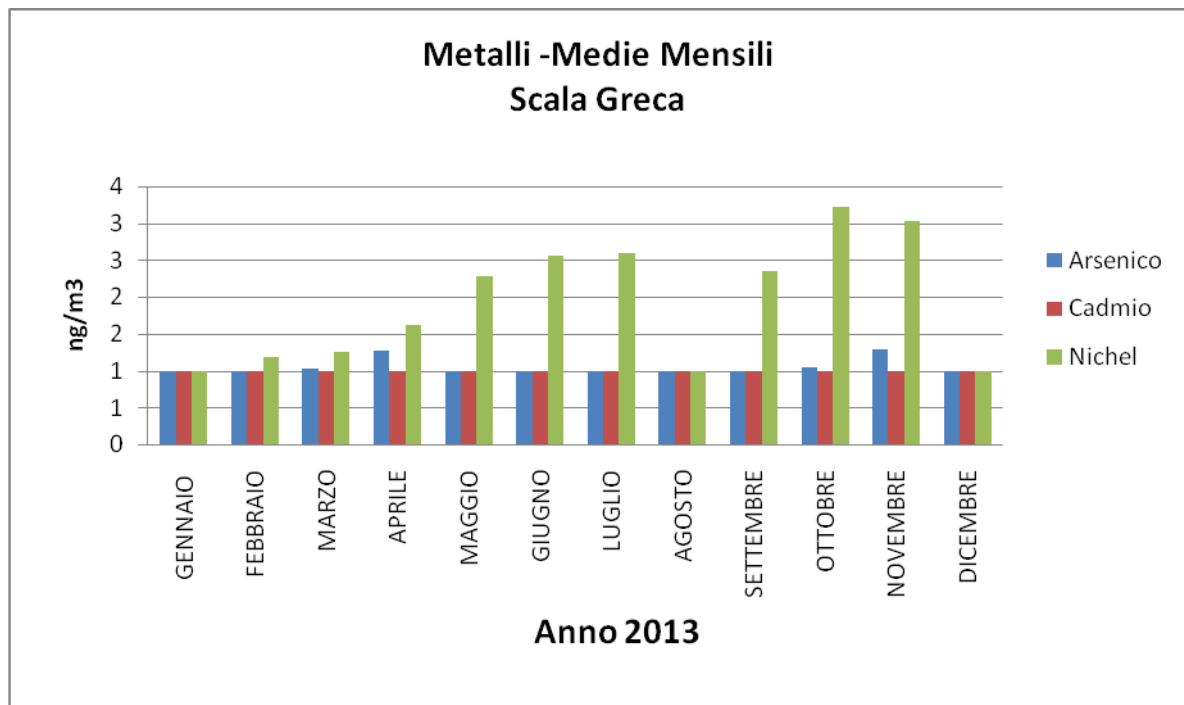
Grafico 22: Metalli- Valore medio mensile
