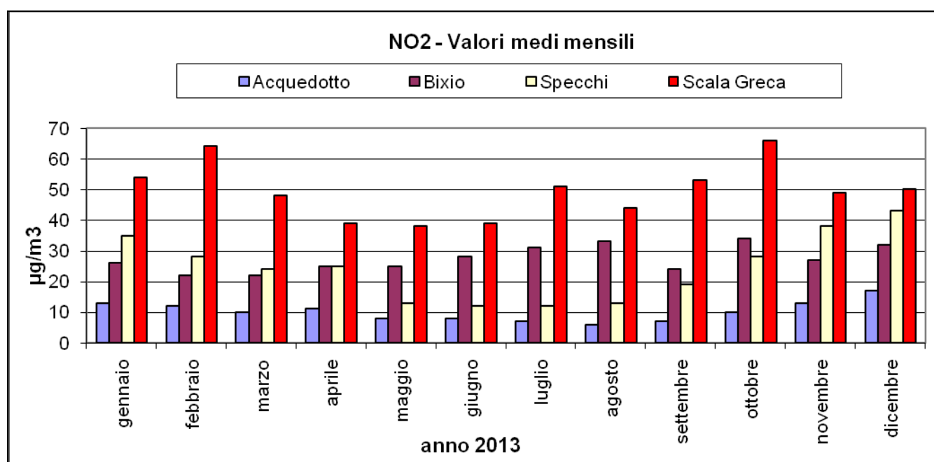
Grafico 10 : NO 2 Valore medio mensile
