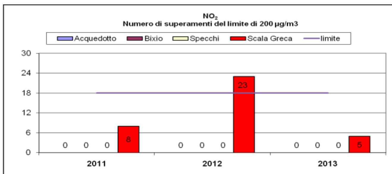
Grafico 8 : NO 2 Numero superamenti del limite orario
