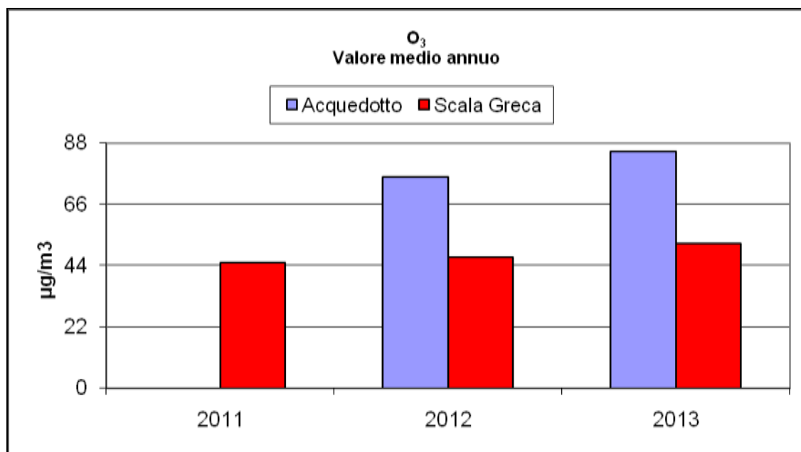
Grafico 15 : O 3 Valore medio annuale
